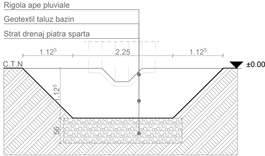
SECȚIUNE TRANSVERSALĂ BAZIN DE CAPTARE APE PLUVIALE SCARA 1:50
