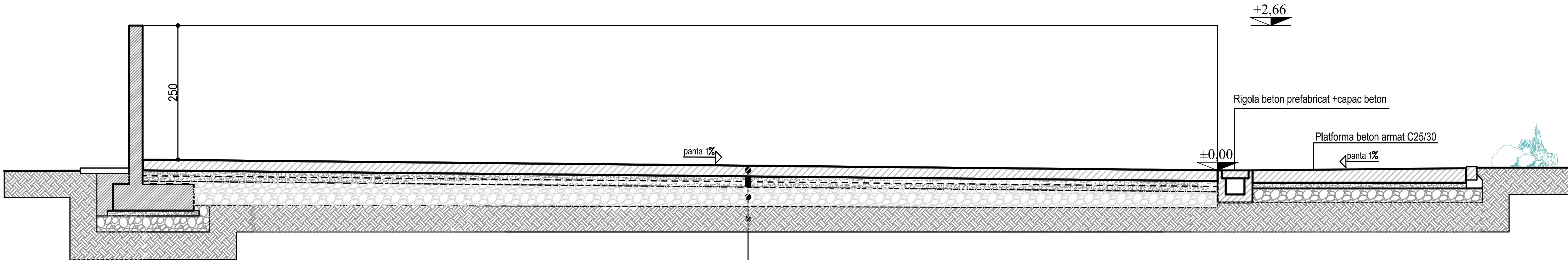
SECȚIUNE TRANSVERSALĂ PLATFORMĂ GUNOI SCARA 1:50
