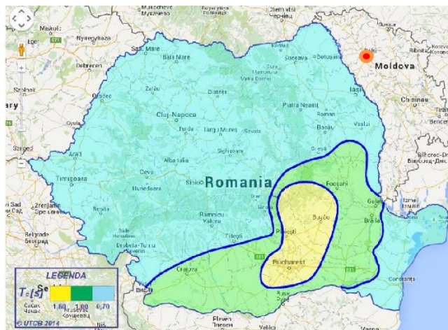
Fig. 2 – Perioada de control (colț) a spectrului de răspuns T_c
