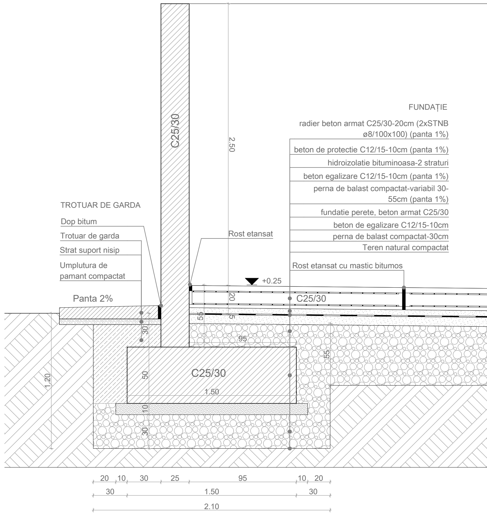
SECȚIUNE FUNDATIE PLATFORMA DE GUNOI SCARA 1:20
